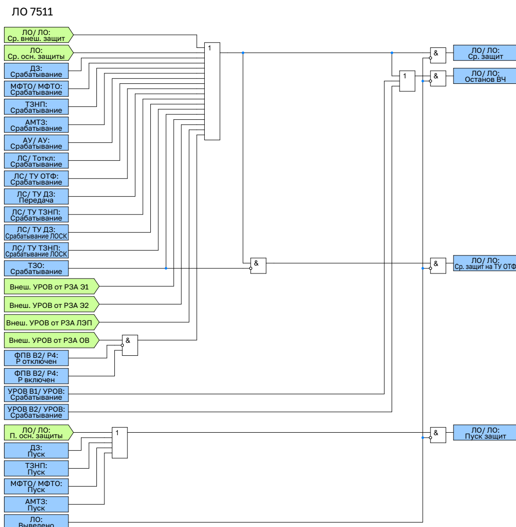
Рисунок 2.77 – Функциональная схема общей логики отключения
